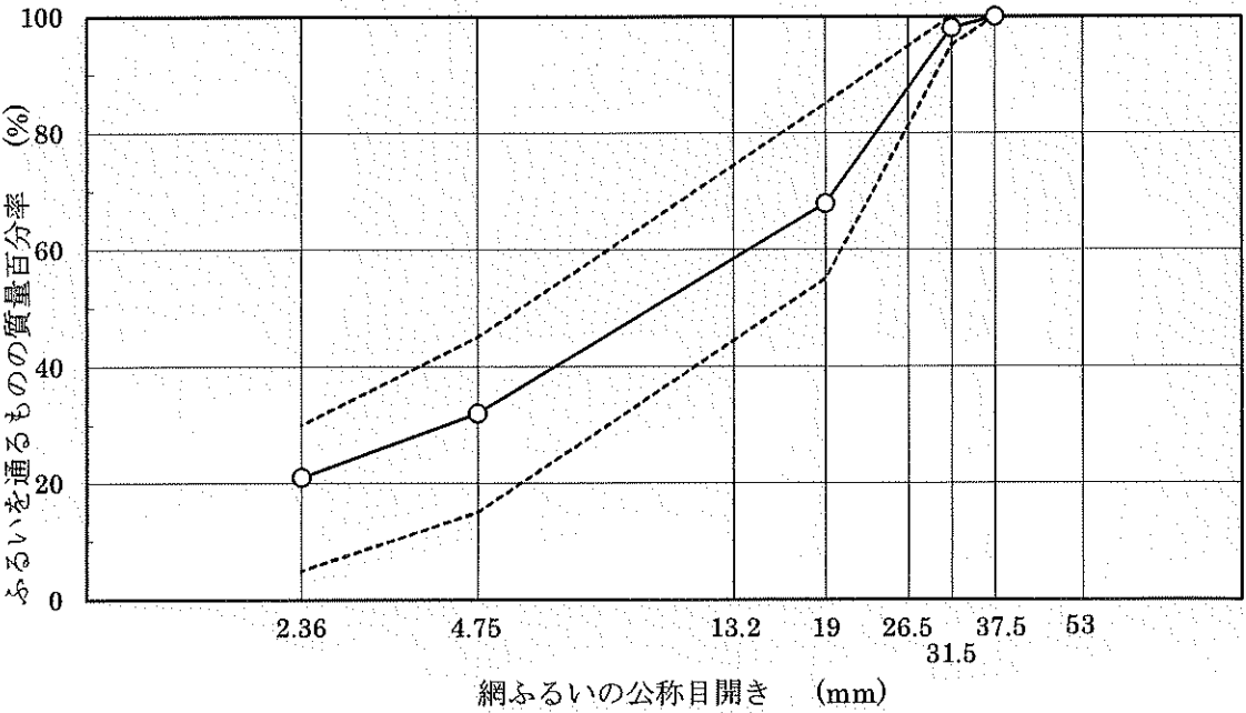
粒 度 曲 線
