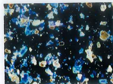
屈折率(1.550) 平行
