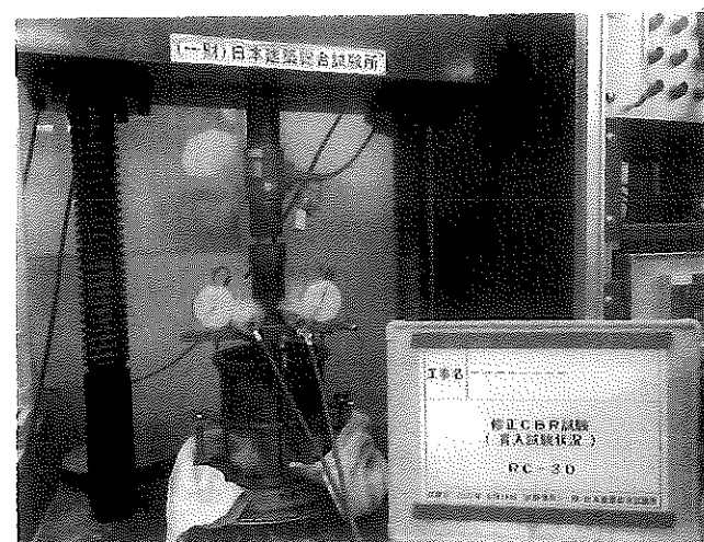
1.8 修正CBR試験 (貫入試験状況)
