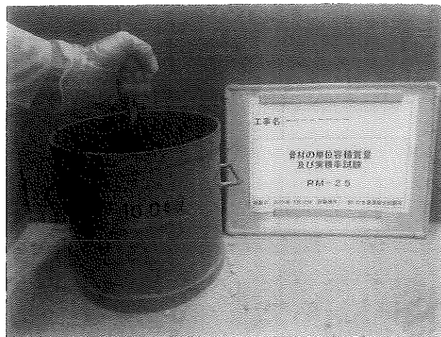
1.2 骨材の単位容積質量及び実積率試験
